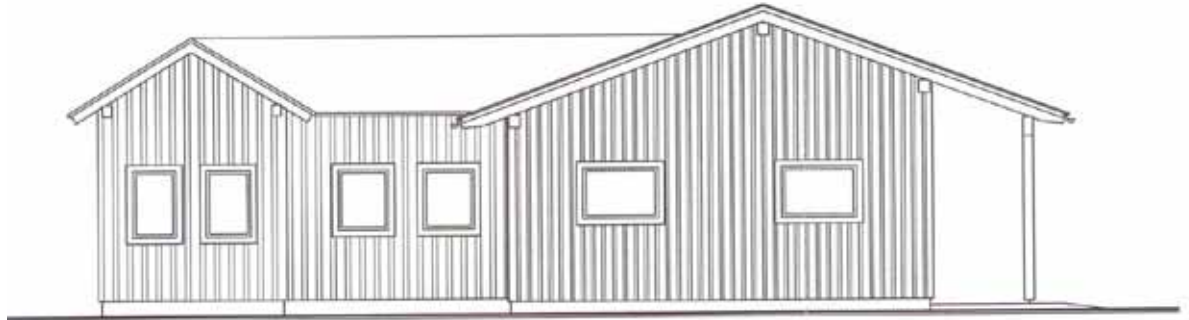
WESTANSICHT
